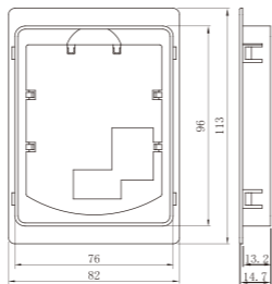
外引键盘卡托安装尺寸 (H*W) : 96×76mm
